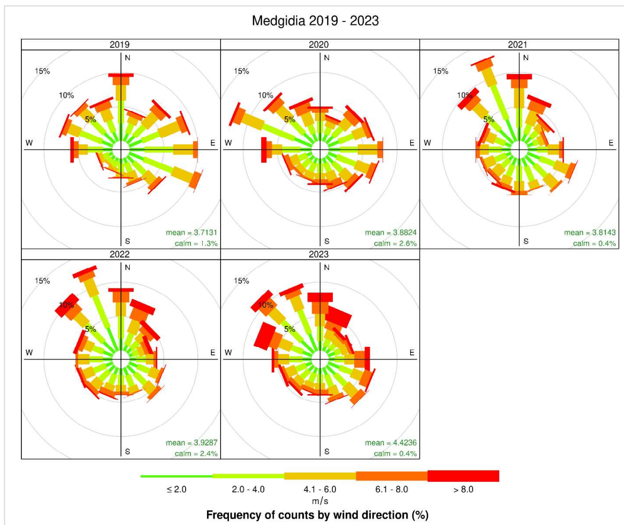
Figura 3-17: Frecvența medie anuală a vântului (%) la stația meteorologică Medgidia în perioada 2019 – 2023
