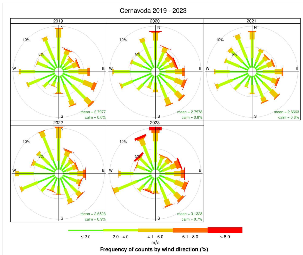
Figura 3-13: Frecvența medie anuală a vântului (%) la stația meteorologică Cernavodă în perioada 2019 – 2023
