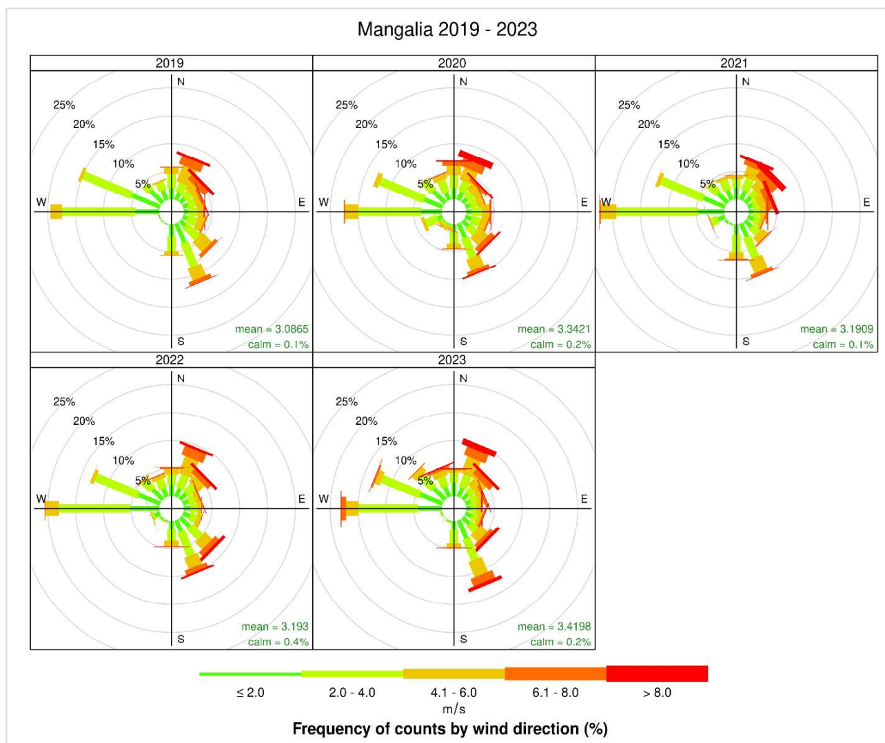
Figura 3-16: Frecvența medie anuală a vântului (%) la stația meteorologică Mangalia în perioada 2019 – 2023
