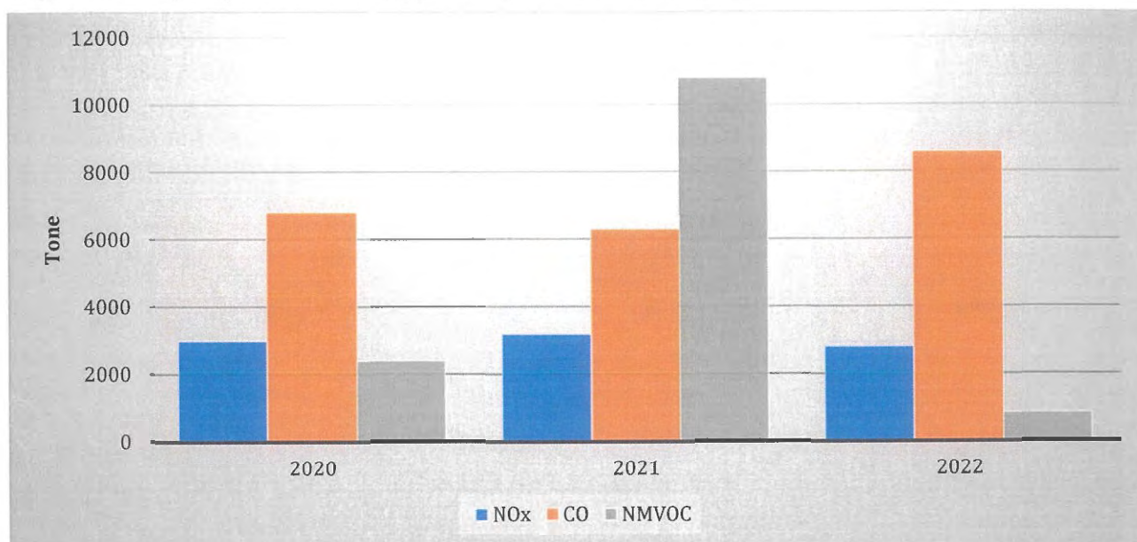
Figura 3-23: Tendința emisiilor totale de poluanți atmosferici precursori ai ozonului (NO x , NMVOC, CO), la nivelul județului Constanța, pentru perioada 2020 – 2022
