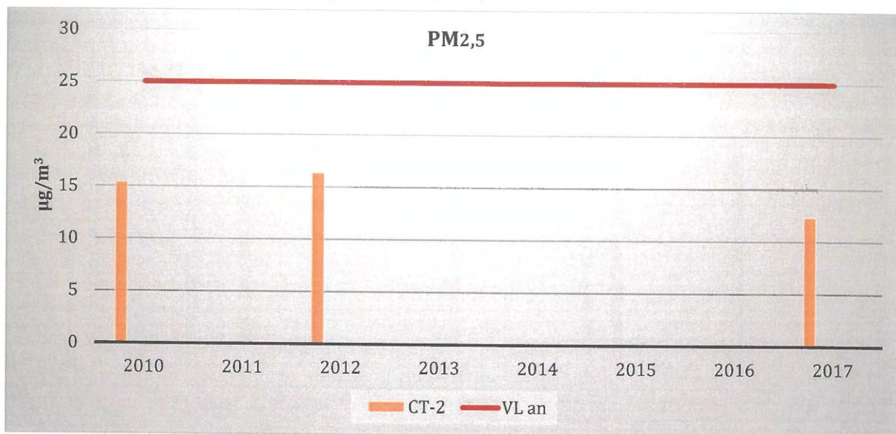
Figura 4-4: Evoluția concentrațiilor medii anuale pentru PM_{2,5} ( \mu g/m^3 ) înregistrate la stațiile automate de monitorizare din județul Constanța în perioada 2010-2017
