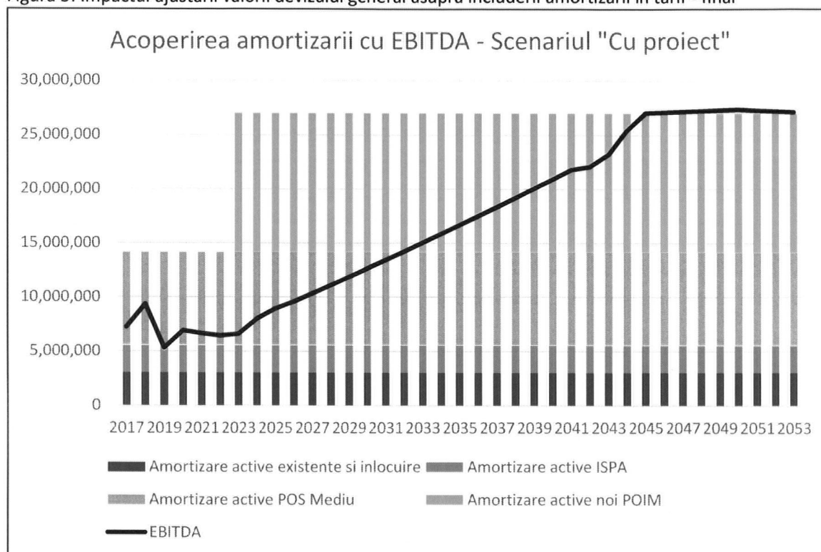
Figura 3: Impactul ajustarii valorii devizului general asupra includerii amortizarii in tarif - final
