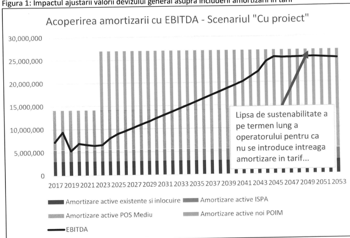
Figura 1: Impactul ajustarii valorii devizului general asupra includerii amortizarii in tarif
